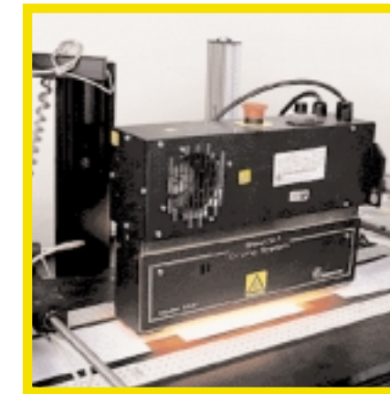
Een hoogvermogen infrarood lamp zorgt desgewenst voor extra droging : zo kunnen ook glanzende substraten feilloos geadresseerd worden.
