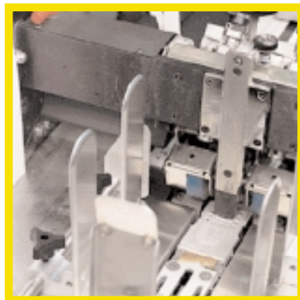
De vacuümshuttle zuigt het onderste exemplaar uit de stapel en geeft het vervolgens door aan de vacuümtransportband : tot 35.000 stuks/uur.
